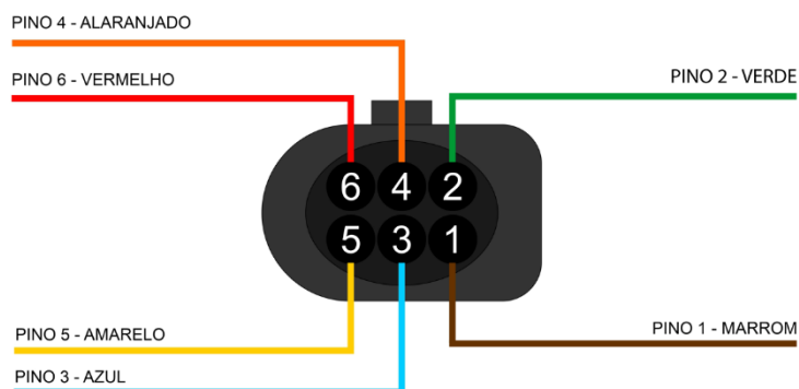
PINOUT SONDA 4.2 (BOSCH)
