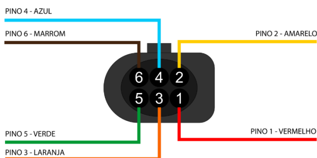
PINOUT SONDA 4.9 (BOSCH)
